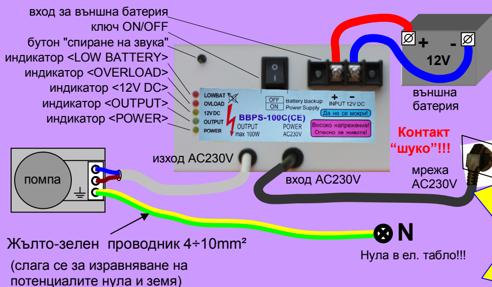
Примерна схема на свързване на аварийен източник BBPS
